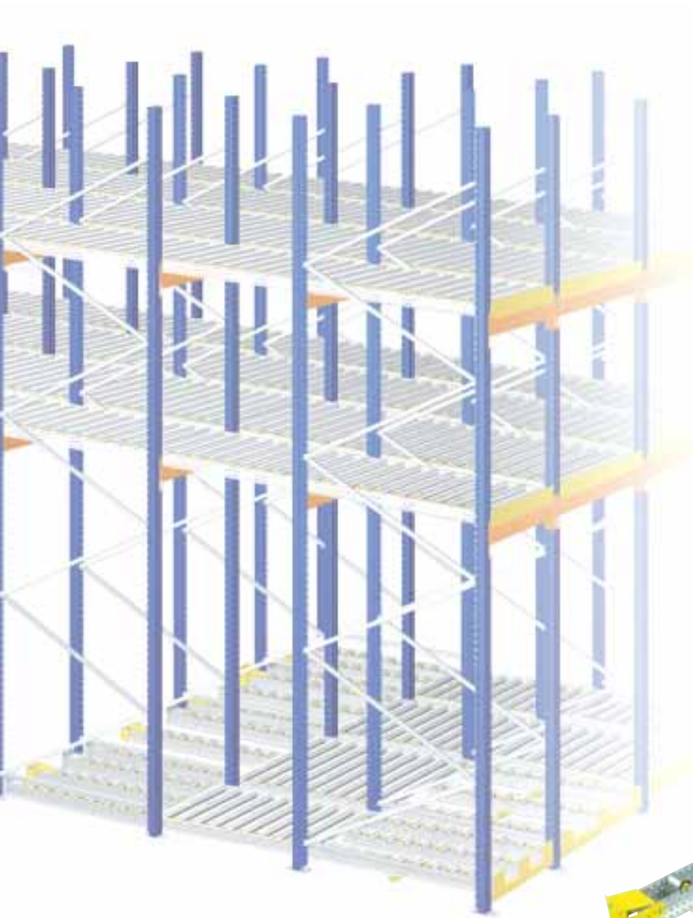
PALLETFLO STP. Gennemløbsbaner hvor udløbsenden er placeret direkte på gulvet. Med udløbsende beregnet til palleløfter.
