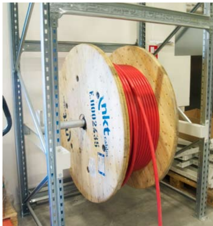
P90 Silverline pallereol er her monteret med beslag til ophæng af kabeltromle.
